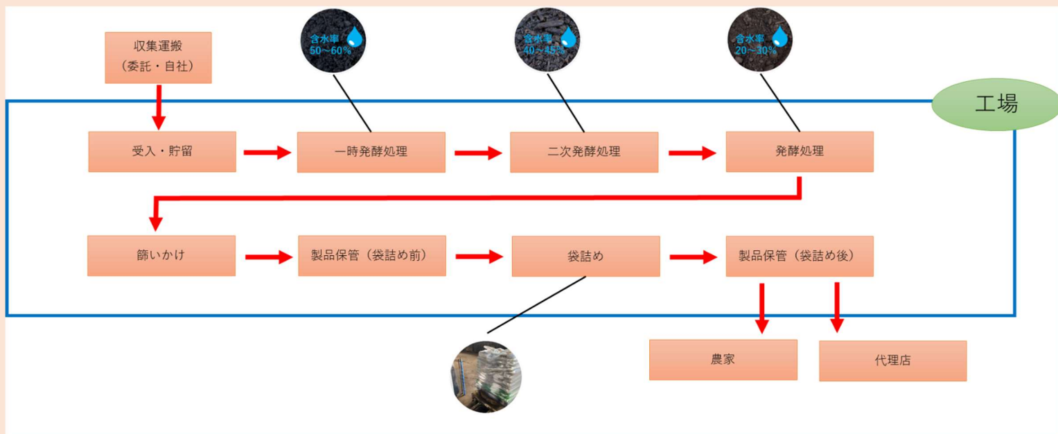
(廃棄物の中間処理・堆肥化フロー図)
